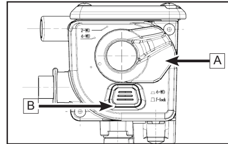
Véhicules sans différentiel arrière
